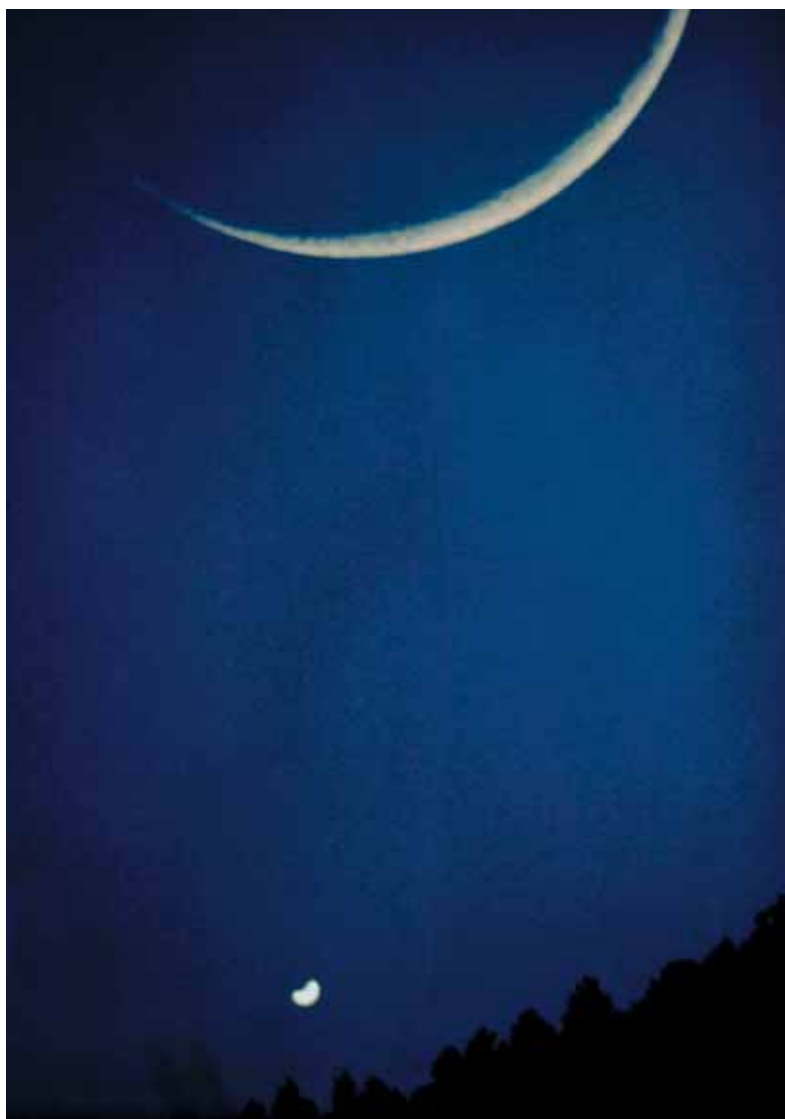
На этой фотографии, полученной 31 декабря 1997 года с телескопа, изображены молодой полумесяц Луны и яркий серп Венеры в раннем вечернем небе города Бурса в Турции
